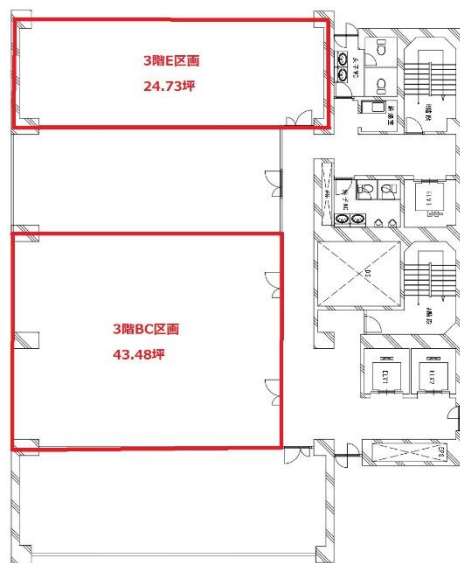
3階
